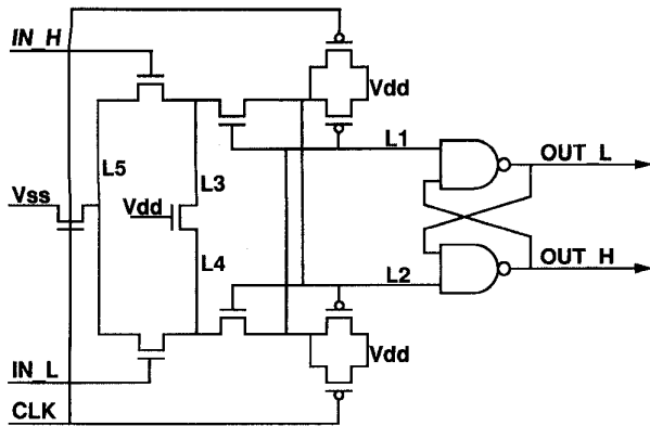
Fig. 11. Latch circuit.
